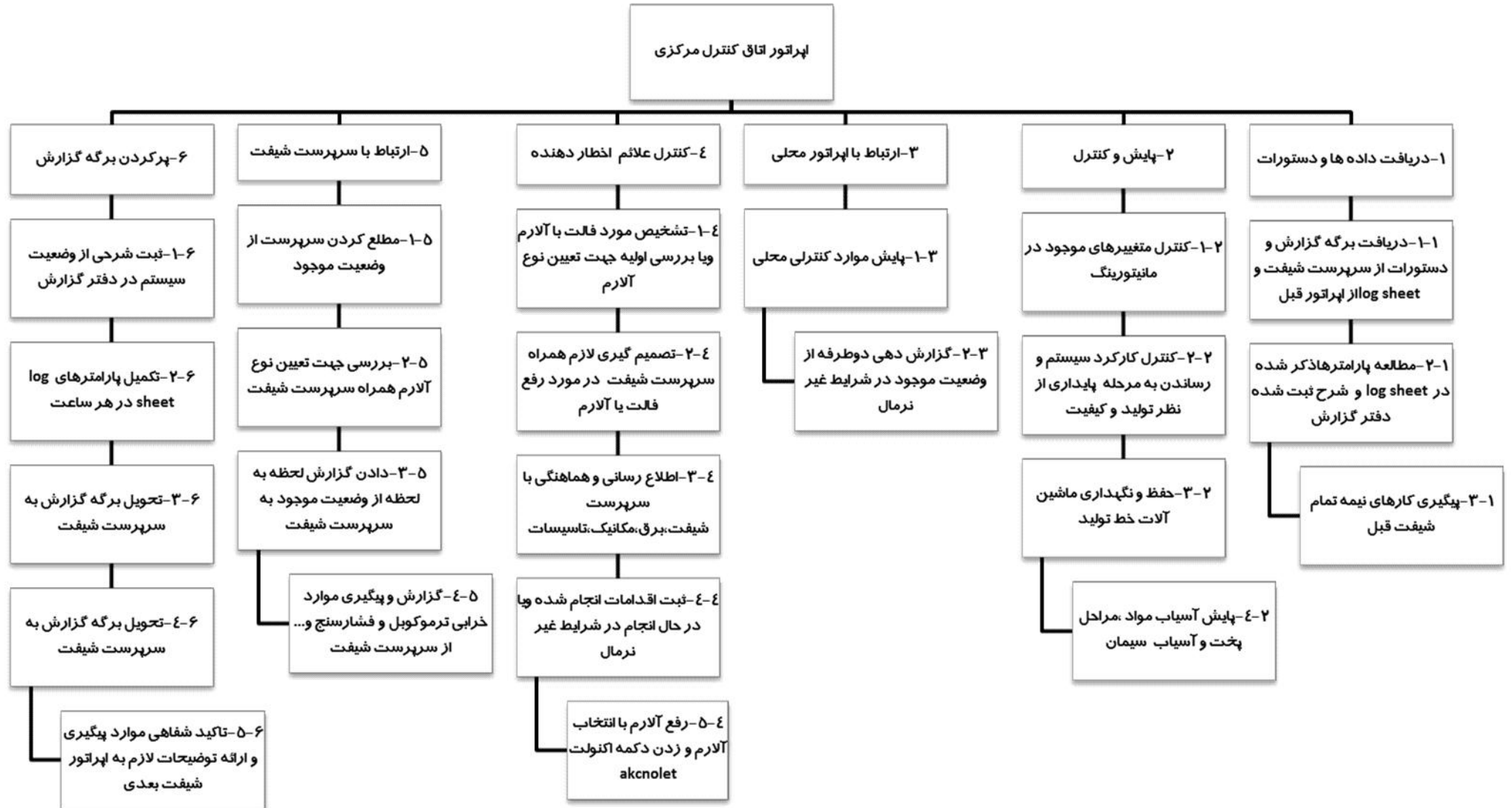
نمودار ۳. آنالیز شغلی به شیوه HTA برای وظایف اپراتور اتاق کنترل مرکزی
